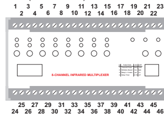
Abb. 1: Klemmen-Nummerierung
