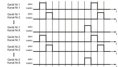
Abb. 4: Funktionsdiagramm Master-Slave-Betrieb
