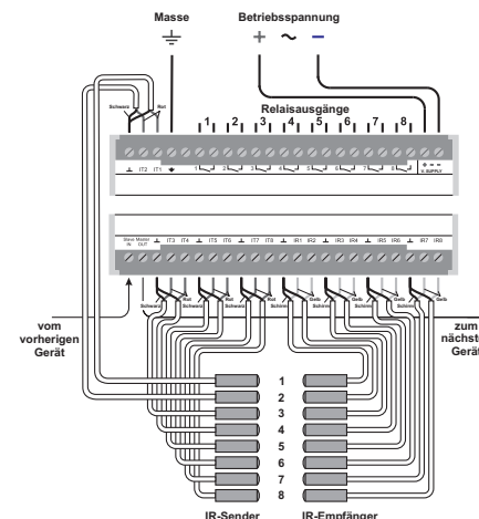
Abb. 2: Anschlussschema
