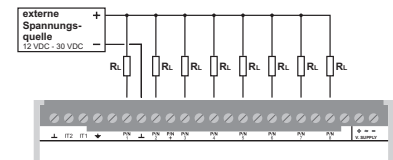
NPN-Schaltung
