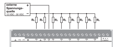
PNP-Schaltung
