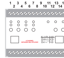
Abb. 1: Klemmen-Nummerierung
