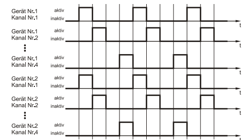
Abb. 4: Funktionsdiagramm Master-Slave-Betrieb
