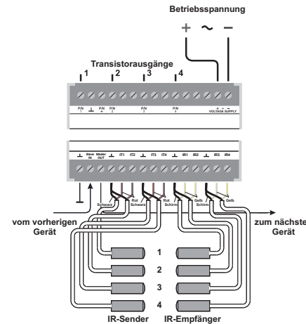
Abb. 2: Anschlussschema
