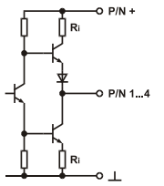
Abb. 3: Transistorausgang
